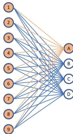
Hình I.8 Ảnh mô tả cách hoạt động của lớp kết nối đầy đủ (fully connected layer)
