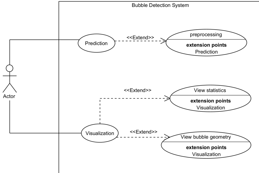
Hình III.7 Usecase tổng quan ứng dụng
