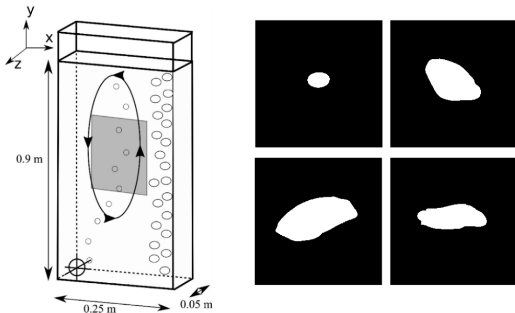
Hình II.2 Hệ thống tạo bọt và ảnh các bọt khí
