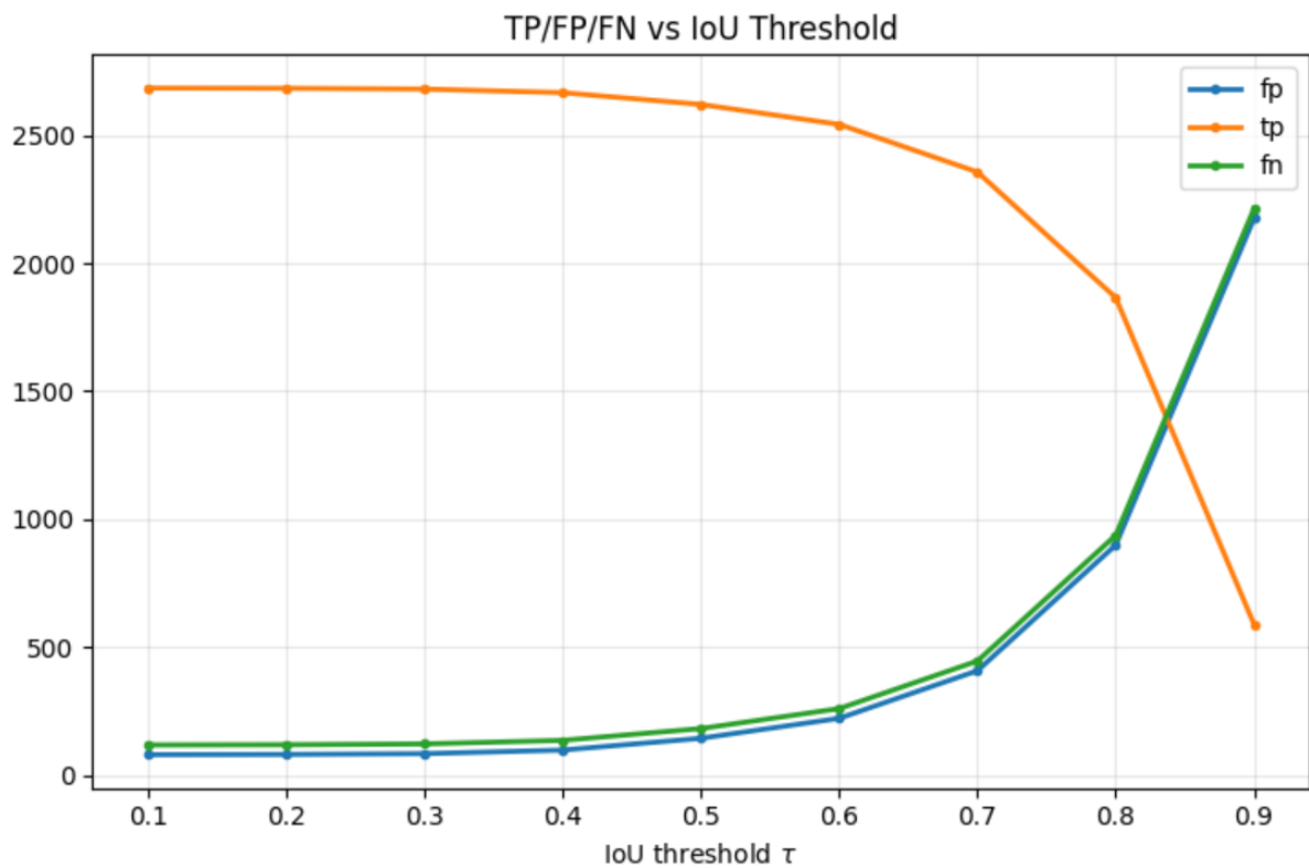
Hình III.2 Tương quan giữa số lượng phát hiện đúng (TP) và sai sót (FP, FN) khi thay đổi ngưỡng đánh giá \tau
