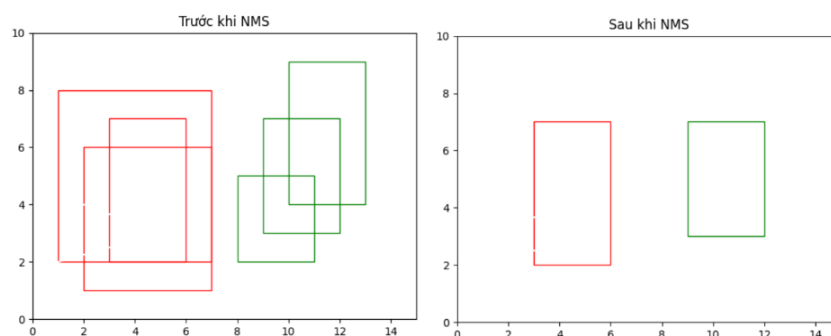
Hình I.12 Minh họa trước và sau khi áp dụng NMS
