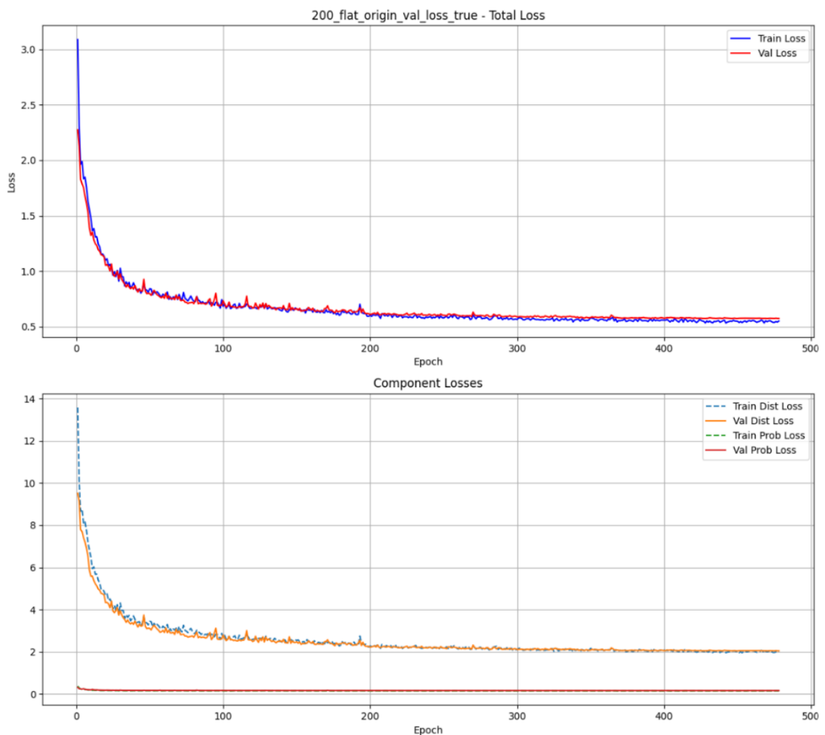
Hình III.3 Biểu đồ các thành phần hàm mất mát
