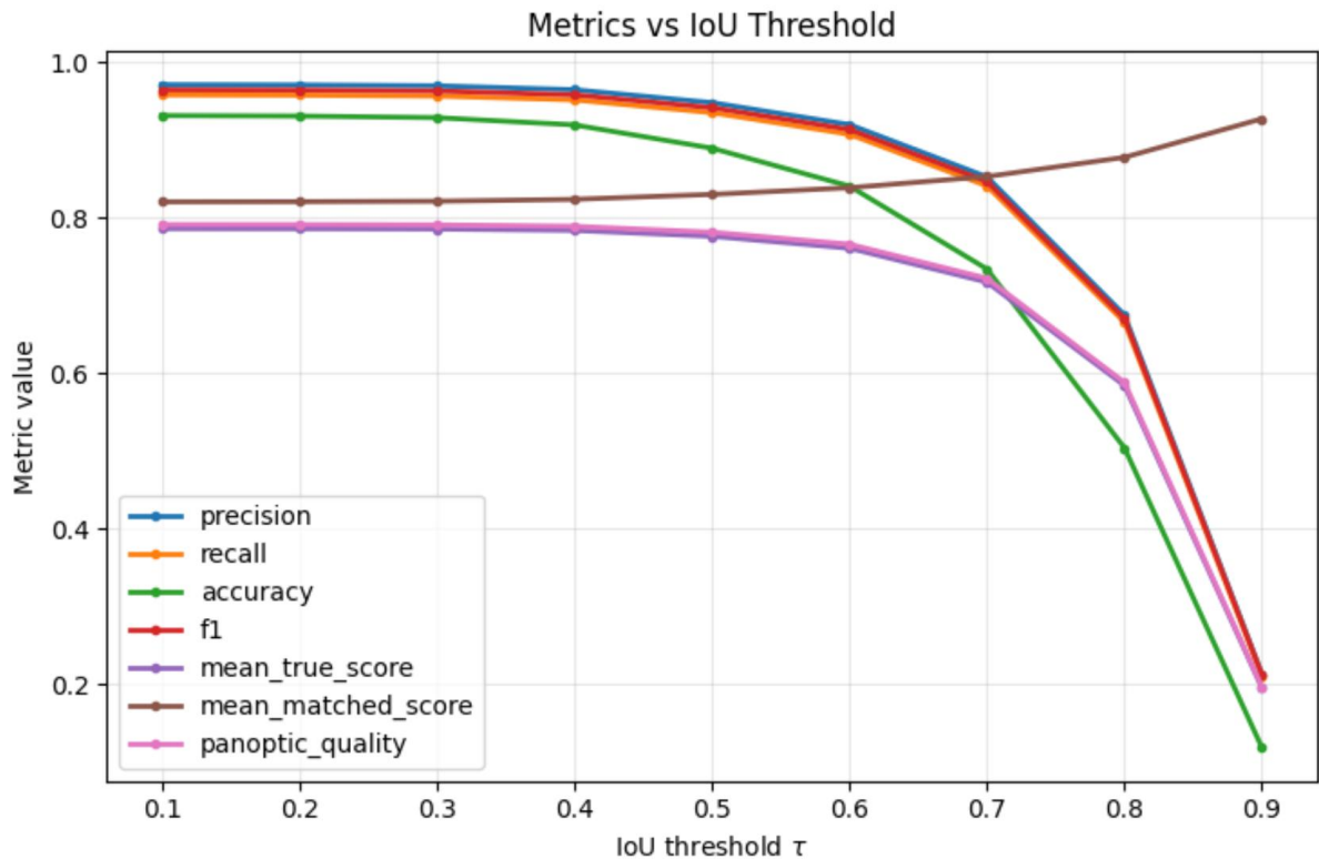
Hình III.1 Sự biến thiên các chỉ số đánh giá của StarDist theo ngưỡng IoU.
