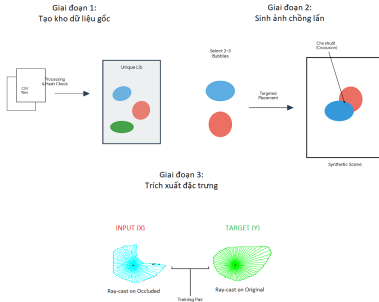
Hình II.8 Các giai đoạn tạo dữ liệu tổng hợp RDC
