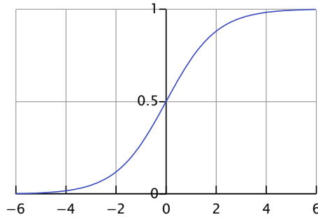
Hình I.10 Ví dụ đồ thị hàm Sigmoid
