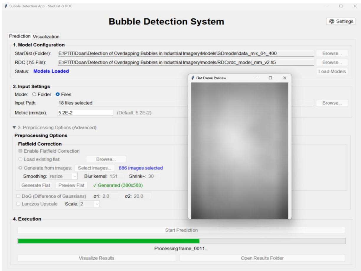
Hình III.9 Giao diện prediction
