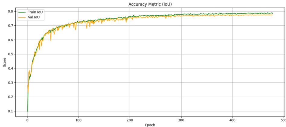
Hình III.4 Biểu đồ IoU
