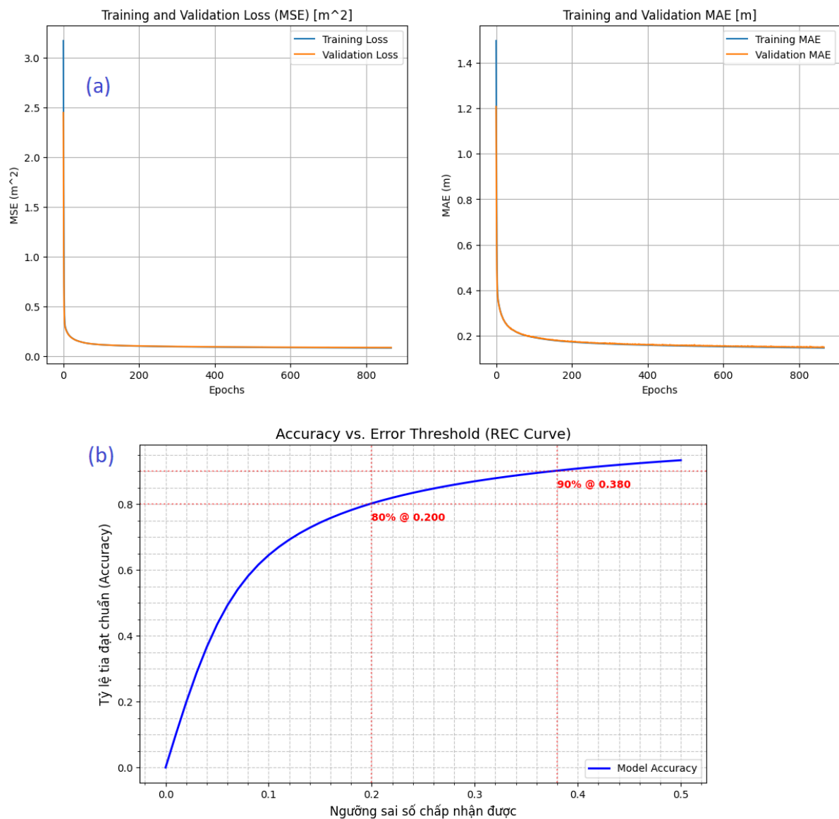
Hình III.6 Phân tích trực quan hiệu năng mô hình RDC
