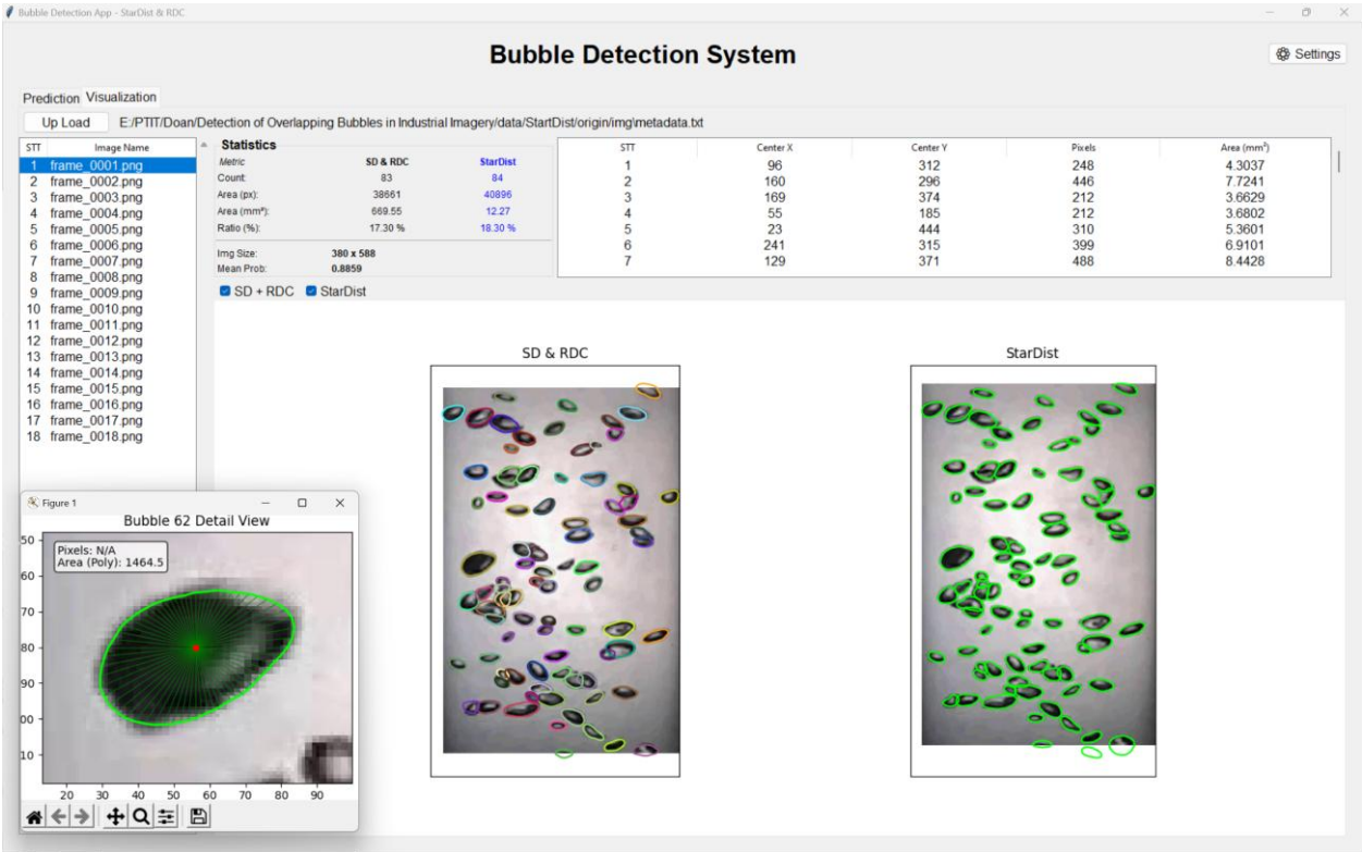
Hình III.10 Giao diện visualization
